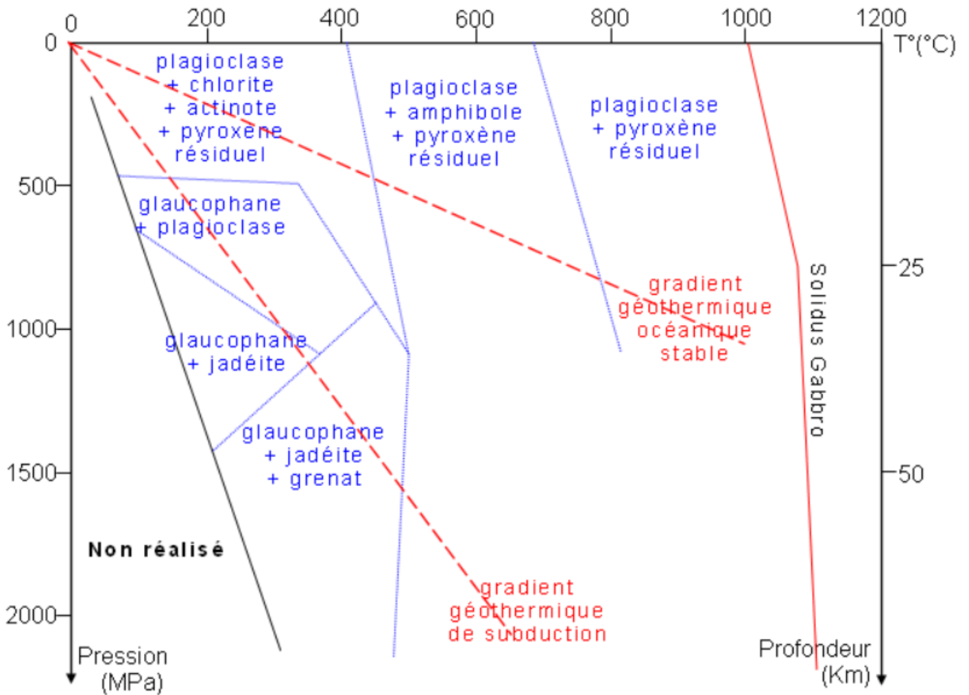
Diagramme de pression et température et faciès métamorphiques
